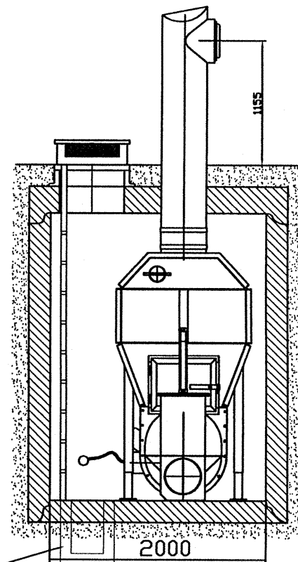
Snit A-A
