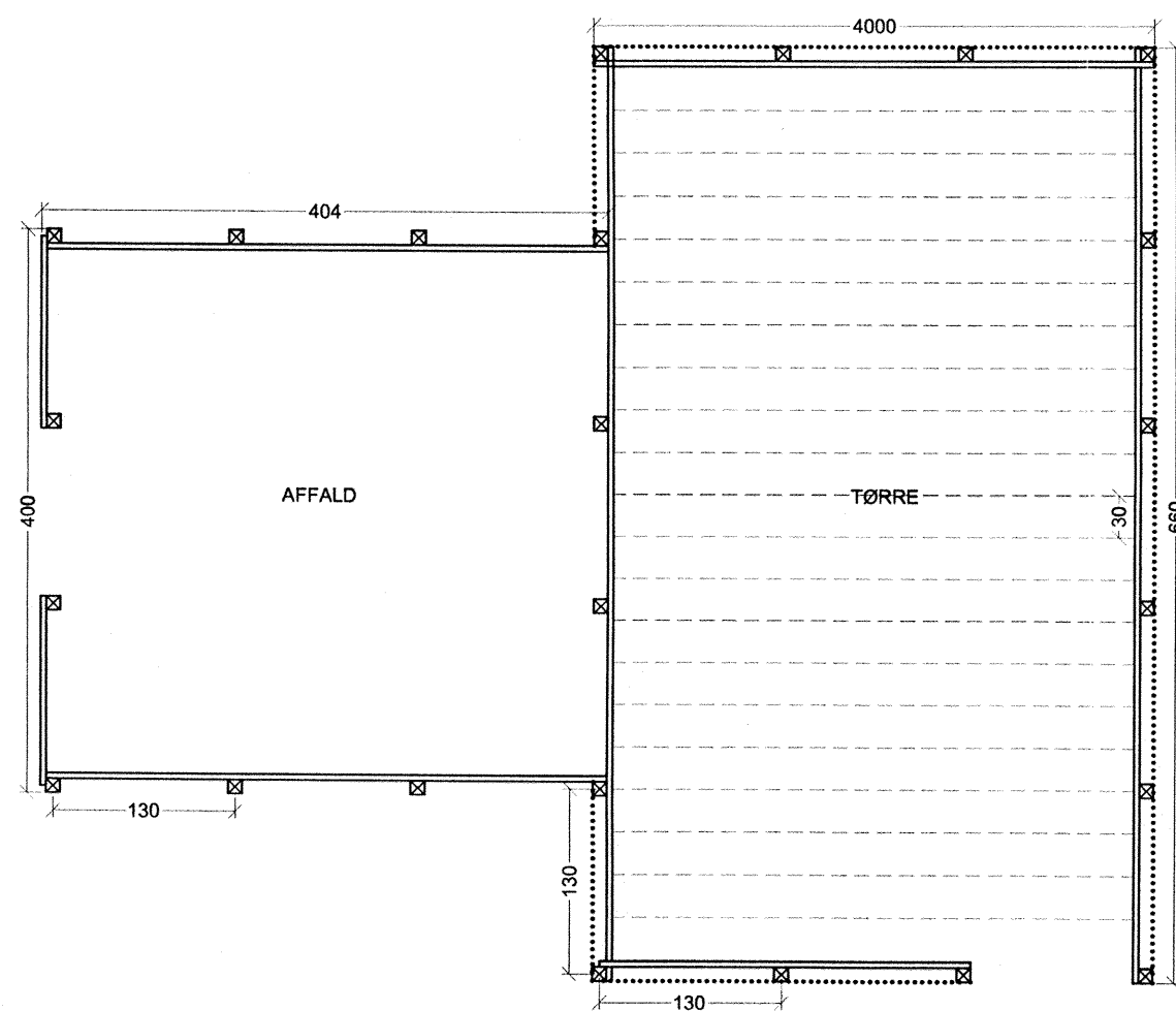
PLAN 1:50, SKURMODUL M1
