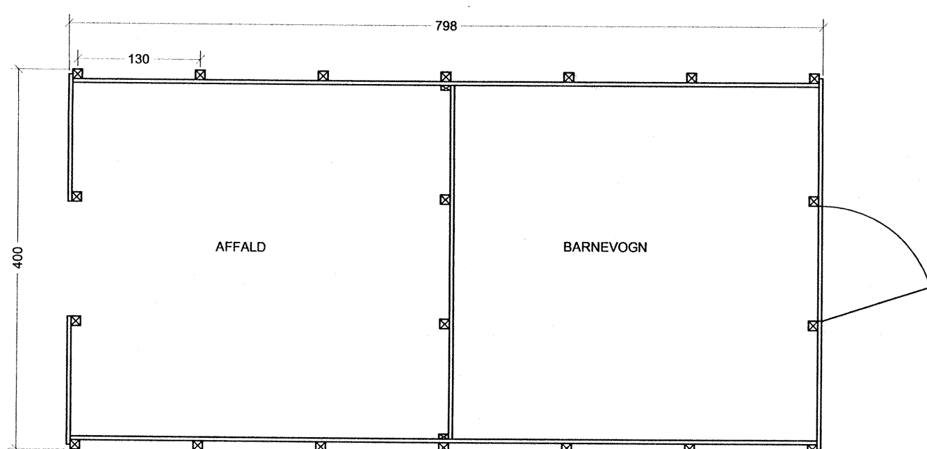
PLAN 1:50, SKURMODUL M4
