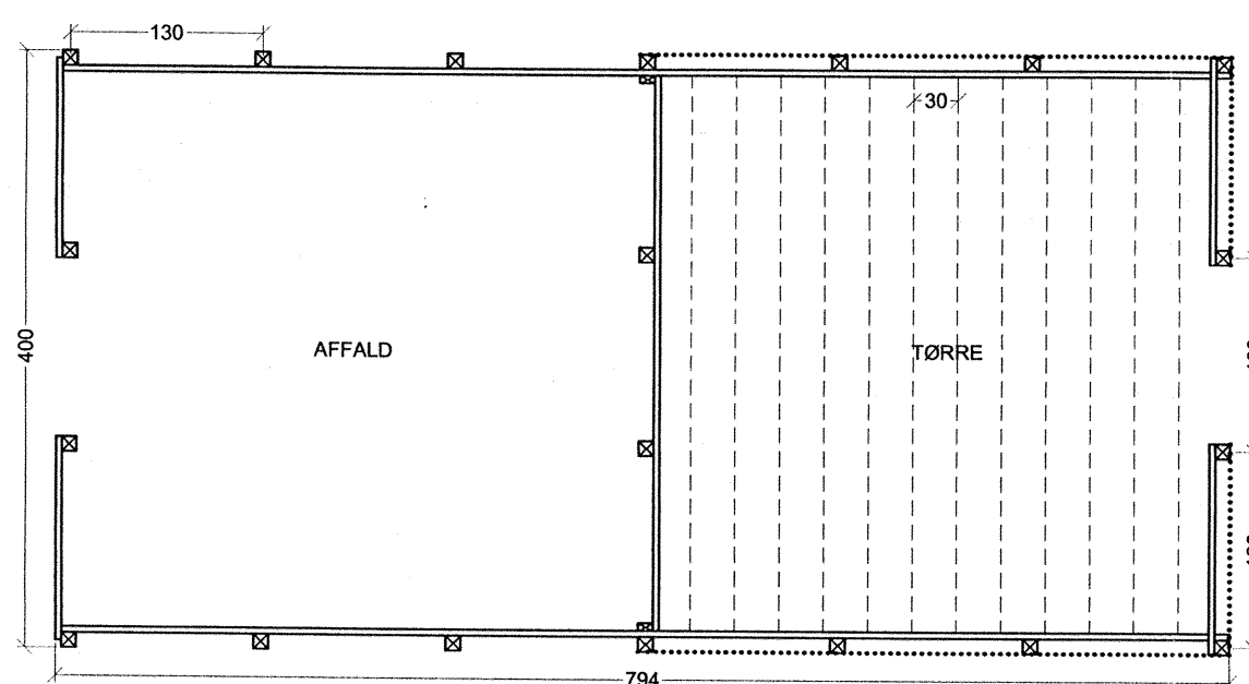
PLAN 1:50, SKURMODUL M2
