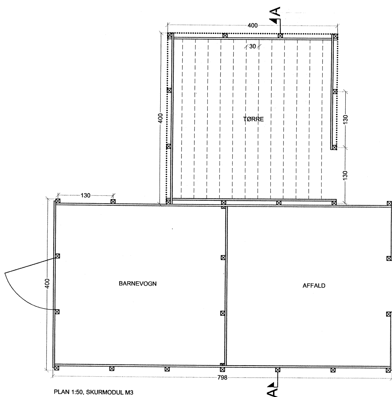
PLAN 1:50, SKURMODUL M3
